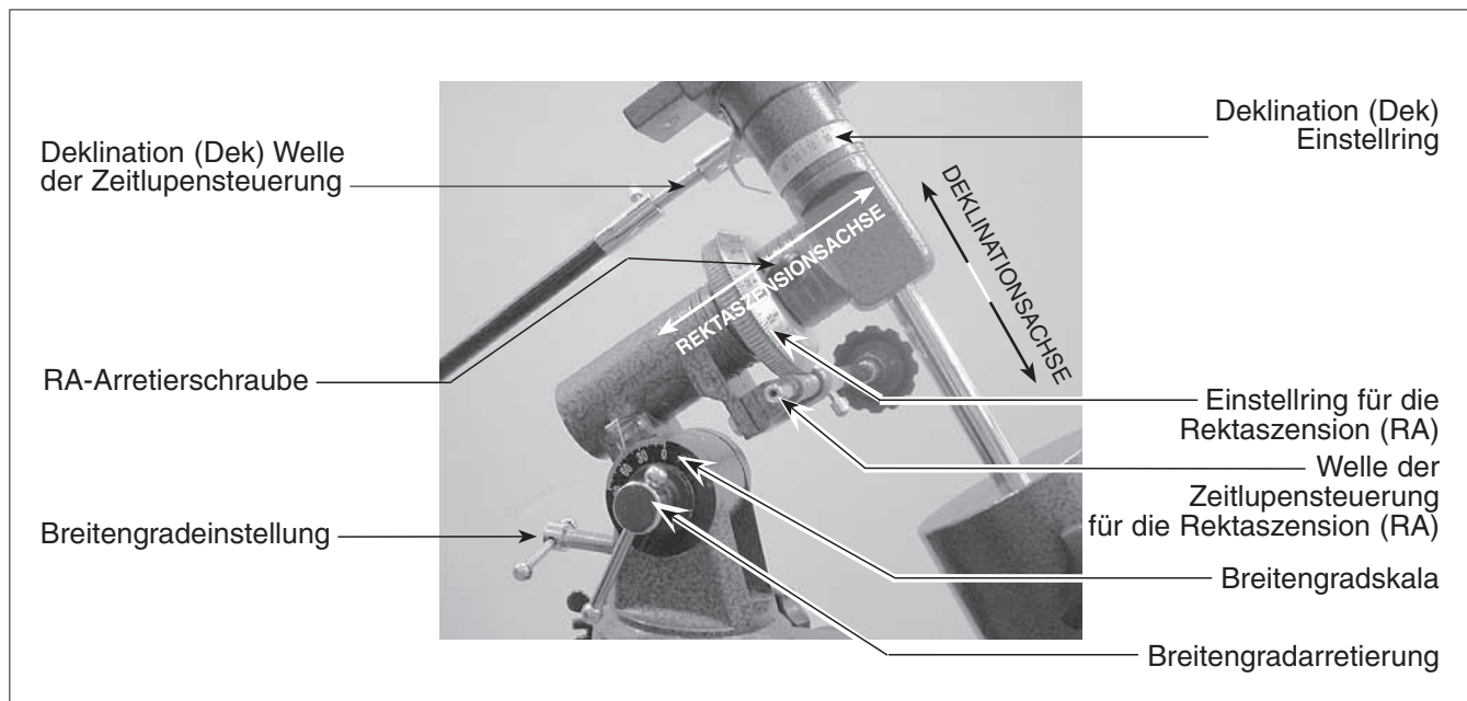
Abbildung 2. Die parallaktische Montierung
