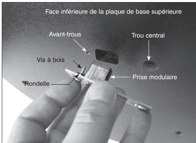
Figure 6. Installez la carte de l'encodeur azimuthal sur la face inférieure de la plaque de base supérieure. Assurez-vous de bien placer une rondelle sur la vis après l'avoir insérée dans le trou de la carte d'azimut, puis vissez-la dans l'avant-trou.
