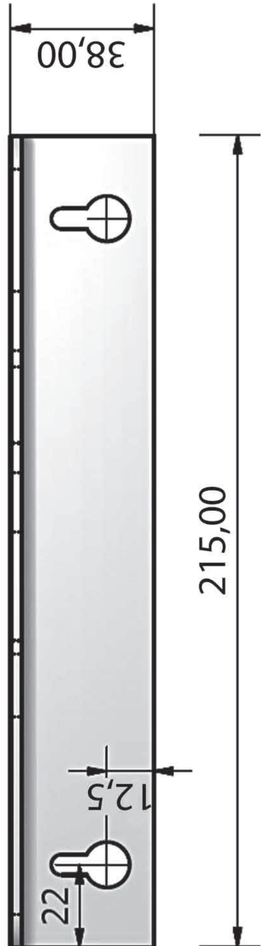
Abbildung 1. Bohrschablone für Schraubenlöcher.
