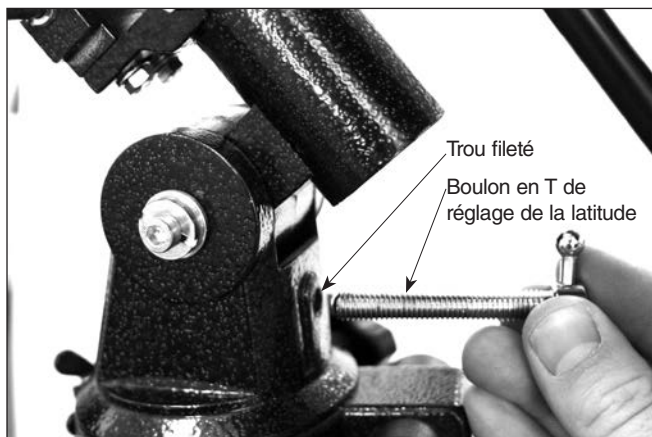
Figure 3. Le boulon en T de réglage de la latitude entre dans le trou fileté situé à l'arrière de la monture.
