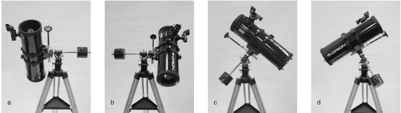
Figure 10. Cette illustration montre le télescope pointé vers les quatre points cardinaux, (a) vers le nord, (b) vers le sud, (c) vers l'est et (d) vers l'ouest. Notez que le trépied et la monture n'ont pas été déplacés. Seul le tube du télescope a été déplacé sur les axes d'ascension droite et de déclinaison.
