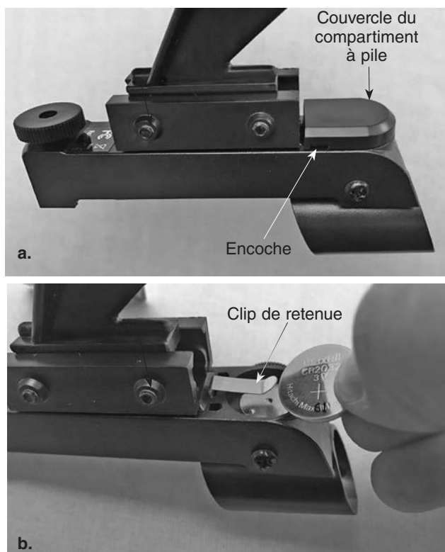
Figure 6. a) Pour installer la pile CR2032 dans l'EZ Finder II, tournez-la à l'envers puis retirez le couvercle du compartiment à pile. b) Installez la pile avec le pôle positif (+) vers le haut, comme illustré.
