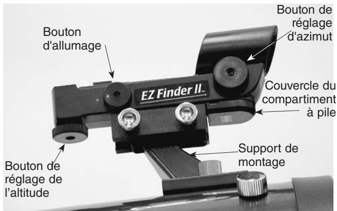
Figure 5. Le chercheur reflex EZ Finder II.
